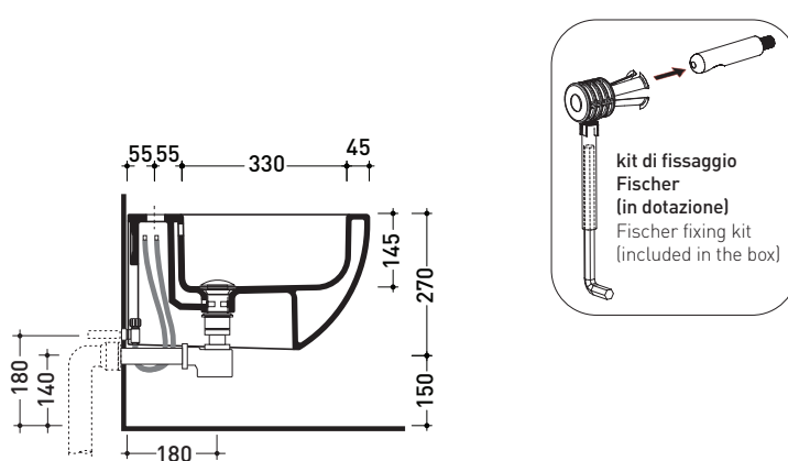
sezione longitudinale / section
