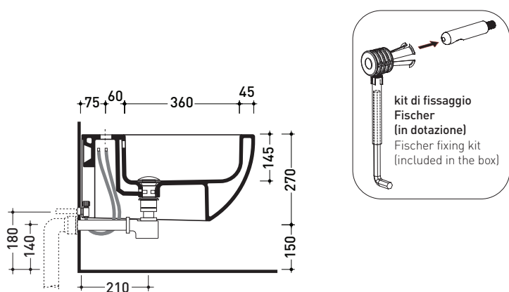
sezione longitudinale / section
