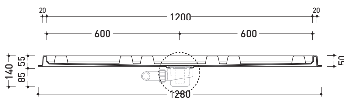
sezione B - B / section B - B
